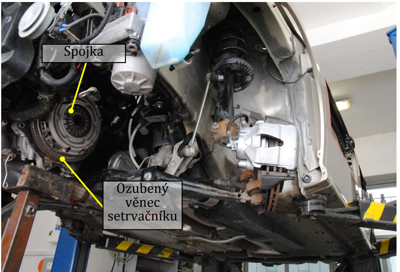
Obr. 4: Pohled pod vozidlo bez převodovky
