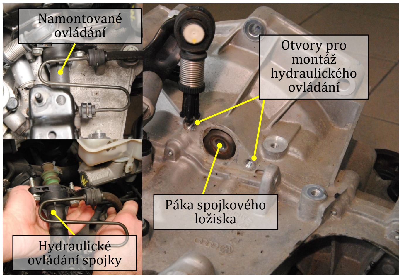
Obr. 15: Montáž hydraulického ovládání spojky
