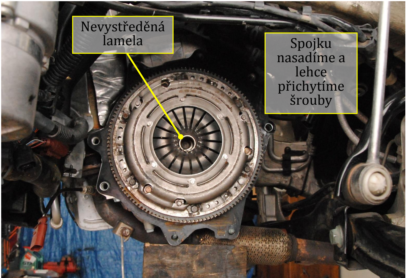
Obr. 10: Montáž spojky
