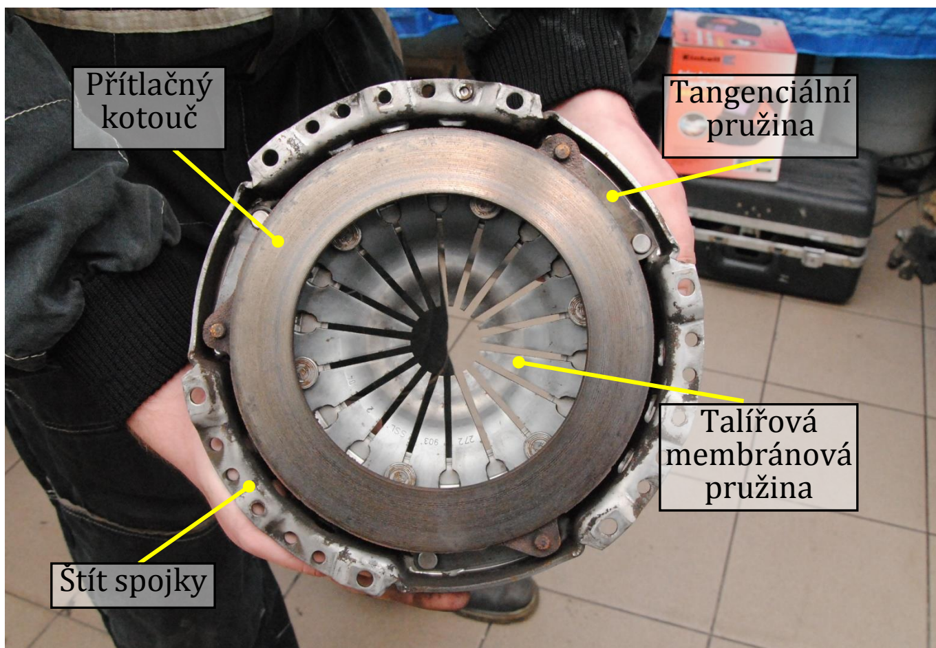
Obr. 8: Štít spojky s pružinou a přítlačným kotoučem
