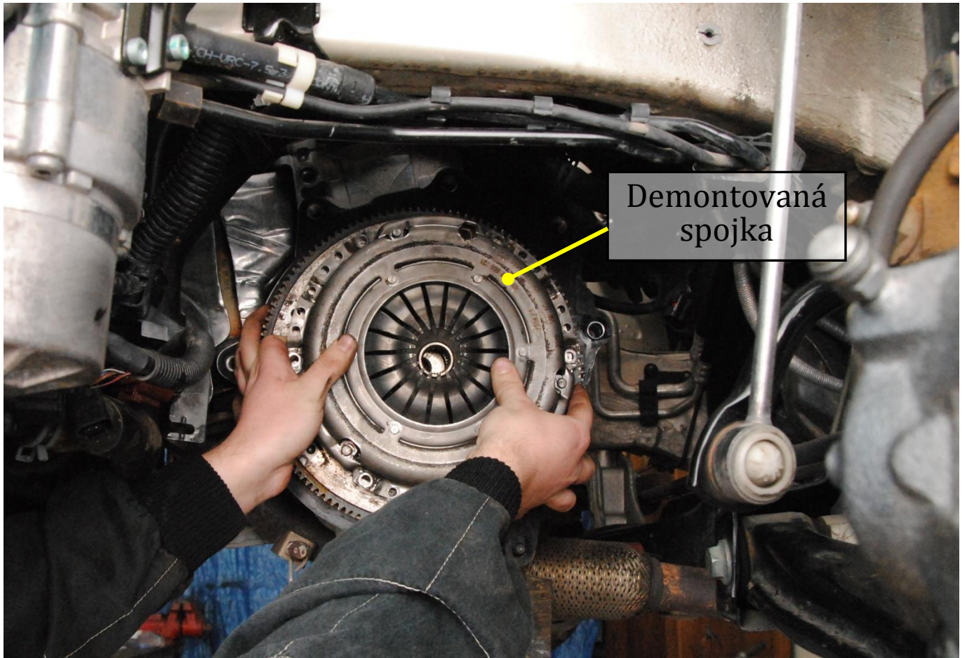
Obr. 6: Demontáž spojky
