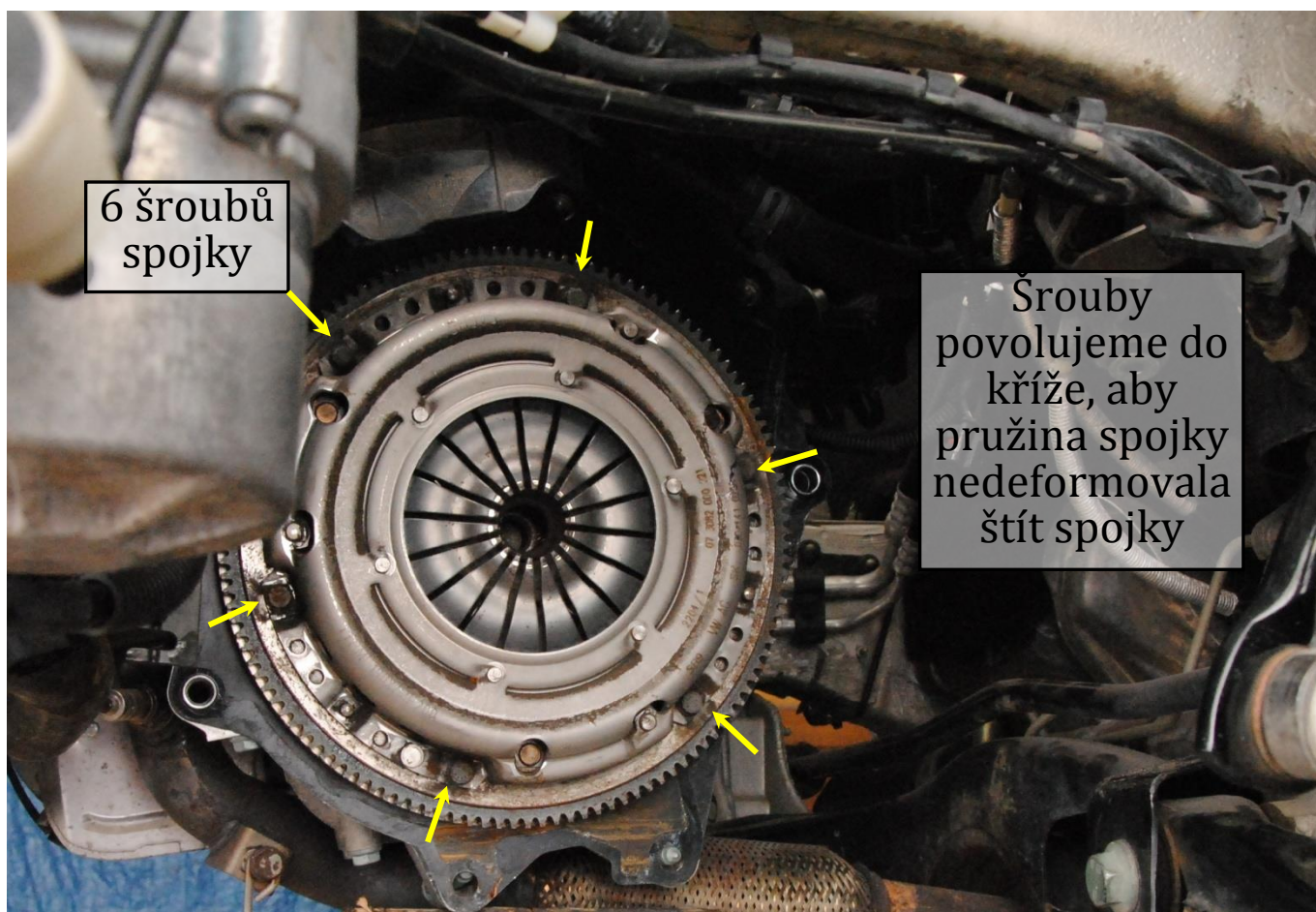
Obr. 5: Demontáž šroubů spojky
