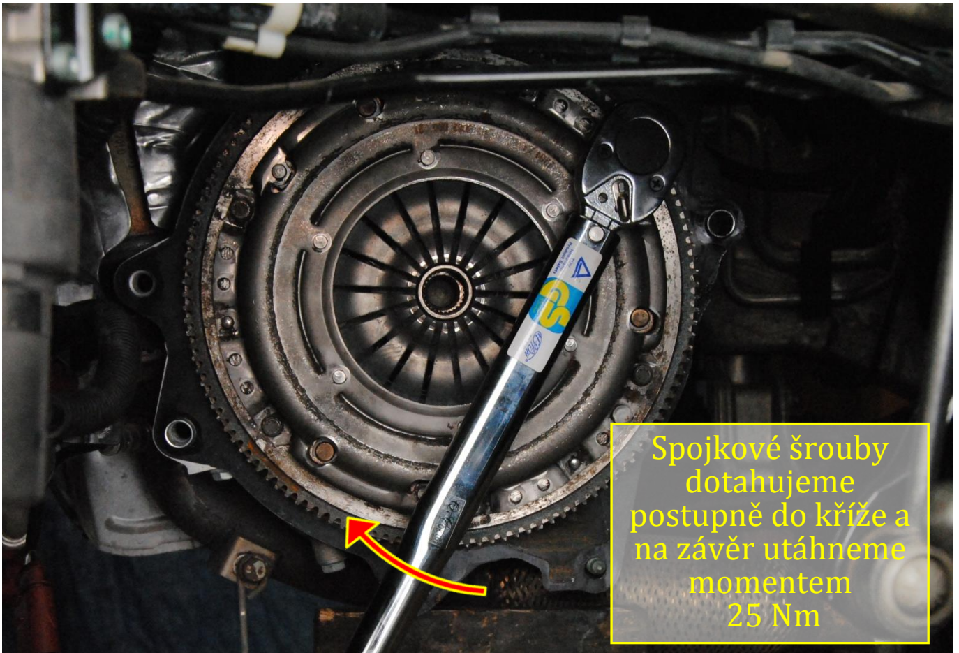
Obr. 13: Dotažení šroubů
