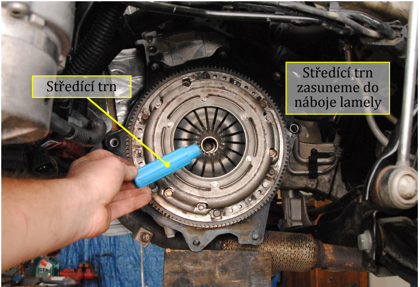
Obr. 11: Vystředění lamely spojky
