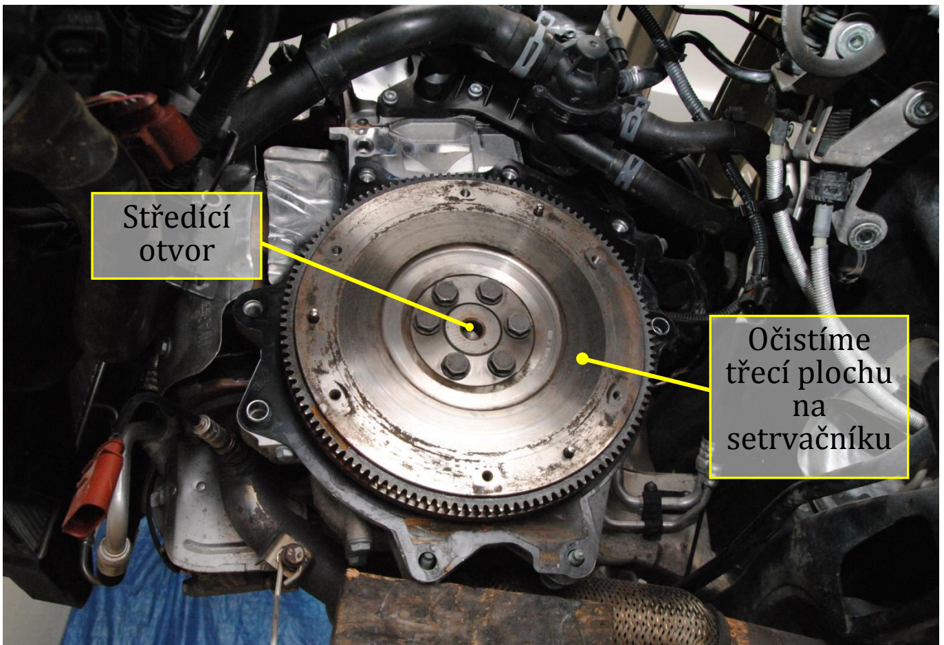
Obr. 9: Setrvačnick motoru
