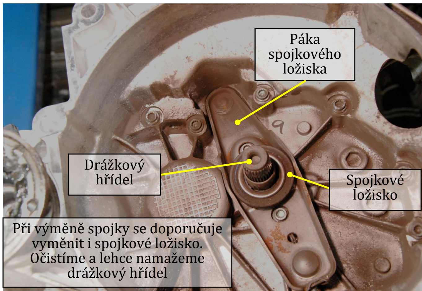
Obr. 14: Vypínací ložisko na převodovce
