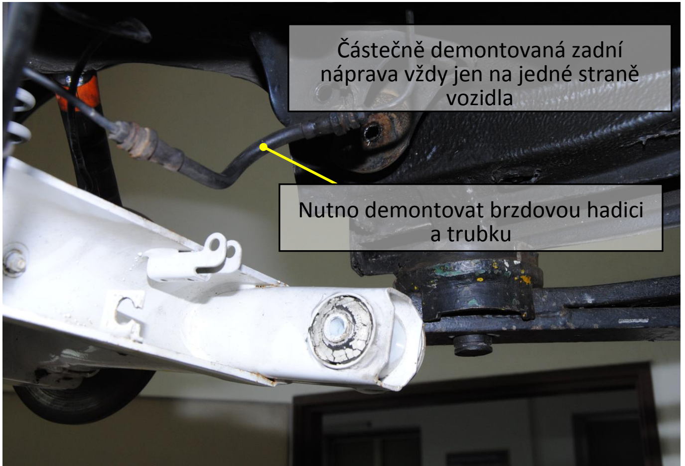
Obr. 8: Částečně demontovaná zadní náprava
