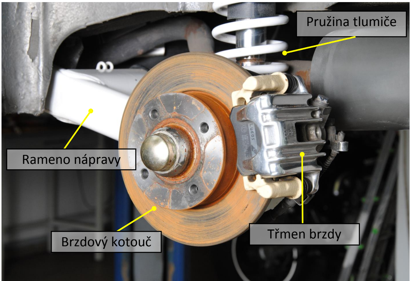
Obr. 6: Detailní pohled na zadní nápravu
