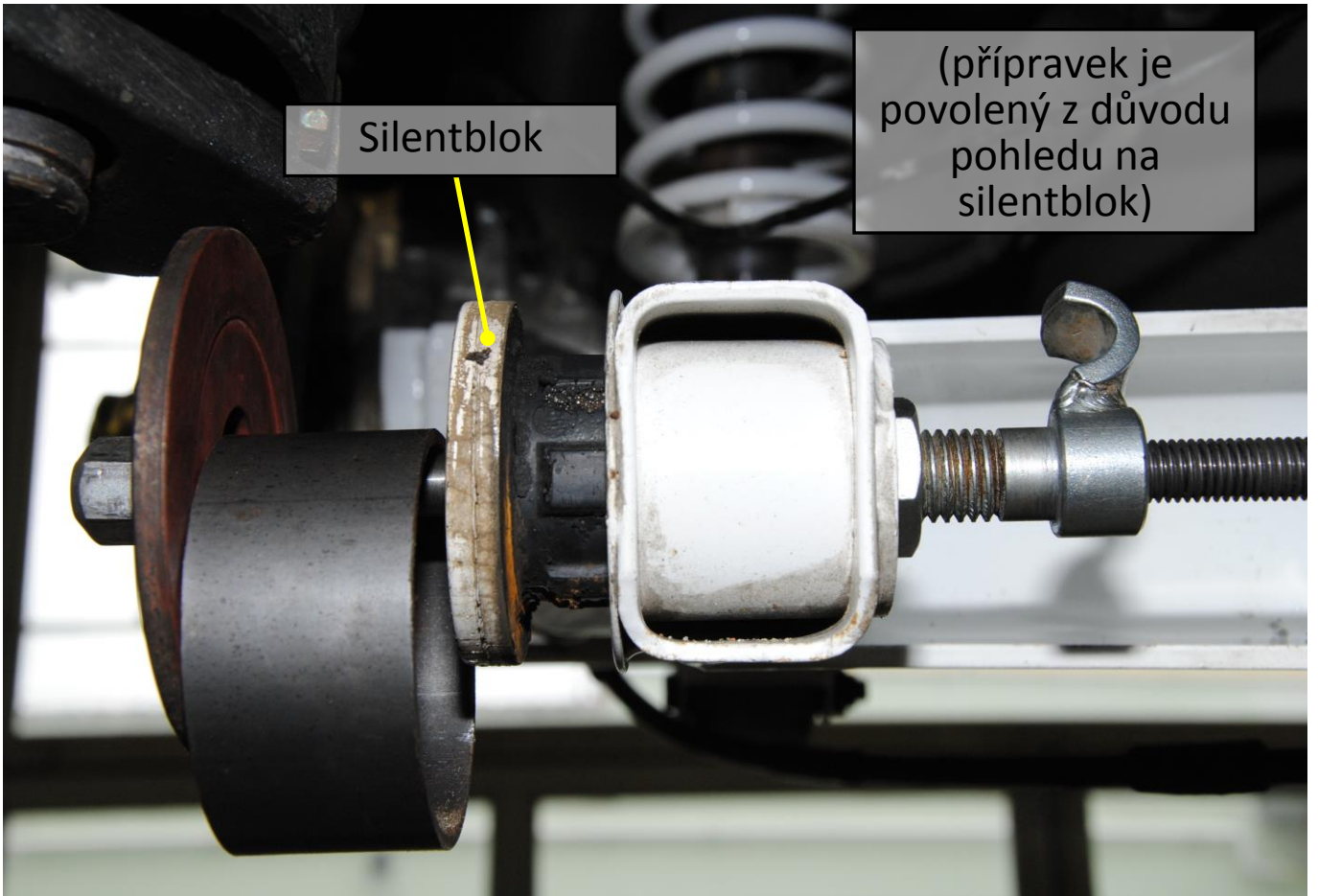
Obr. 10: Částečně vylisovaný silentblok
