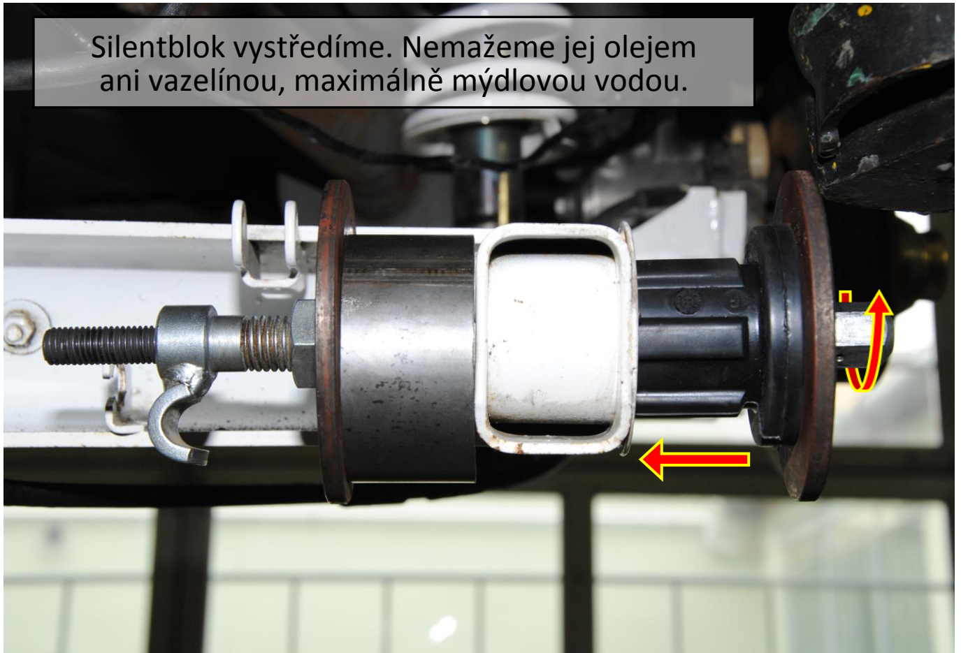
Obr. 16: Vystředění silentbloku a jeho lisování
