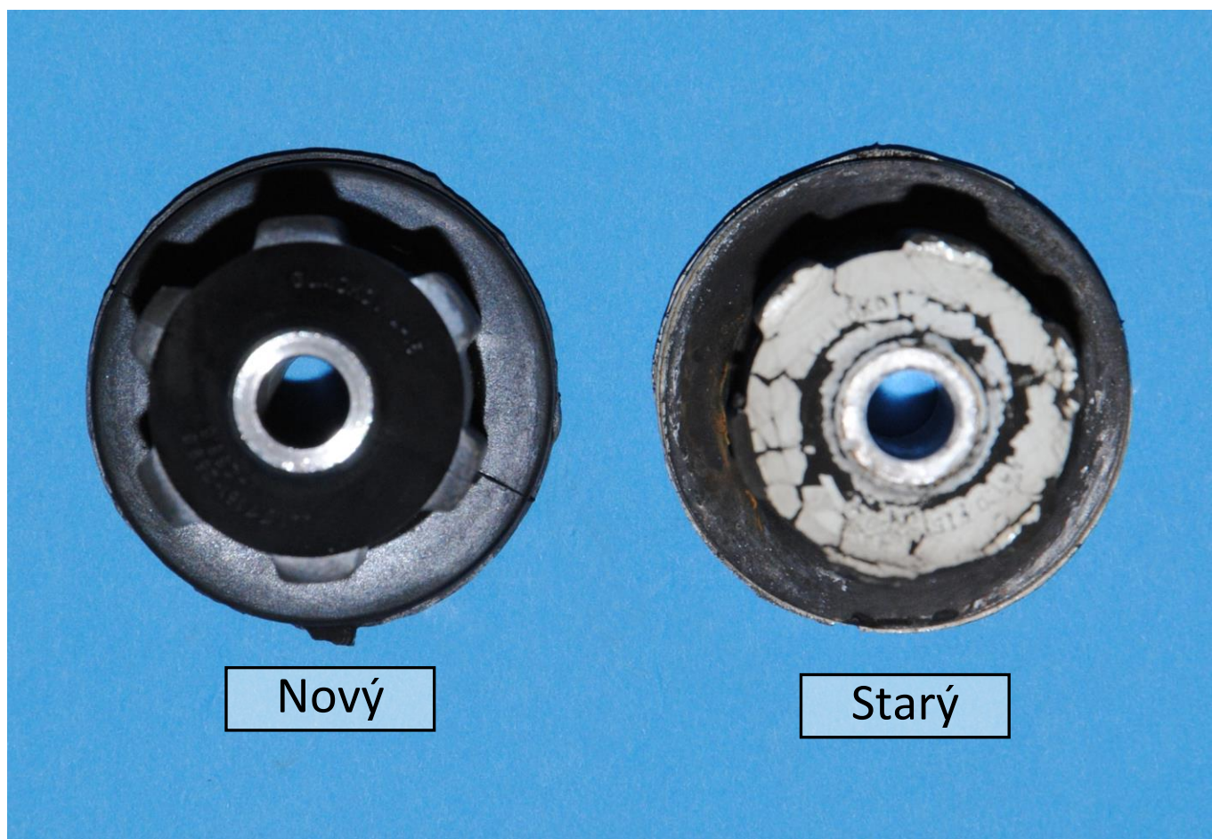
Obr. 12: Porovnání silentbloků
