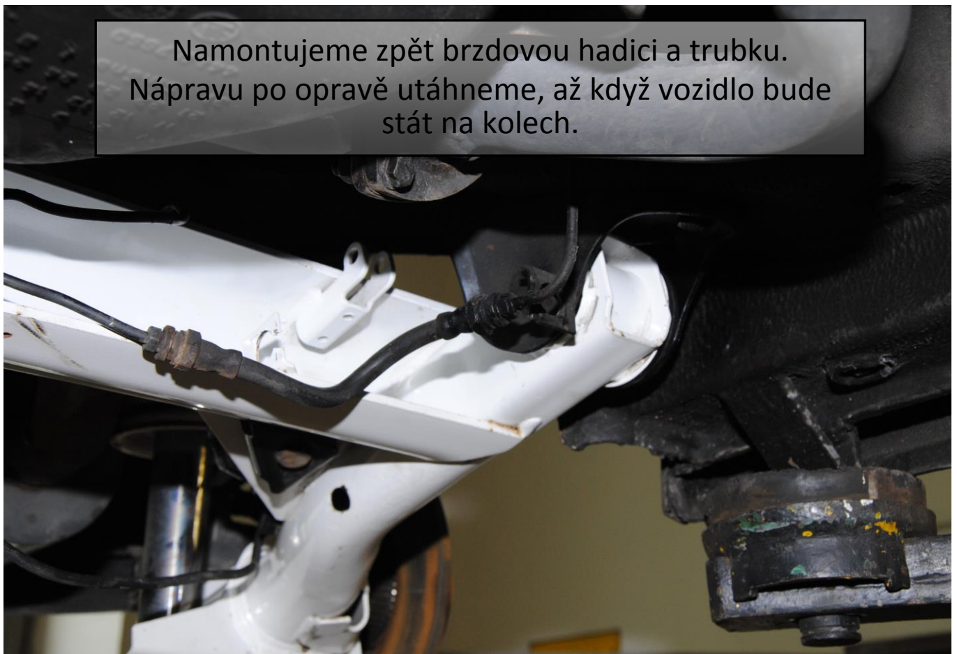
Obr. 18: Zpětné uchycení nápravy do oka karoserie
