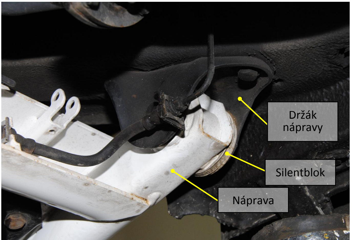
Obr. 7: Pohled na uložení zadní nápravy (přes silentblok do karoserie)
