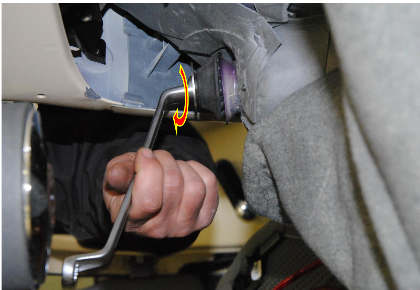
Obr. 25: Dotažení zajišťovací matice
