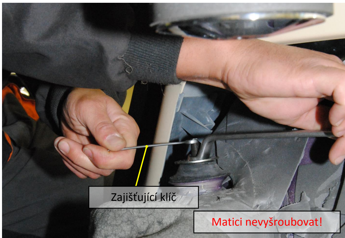
Obr. 4: Povolení zajišťovací matice
