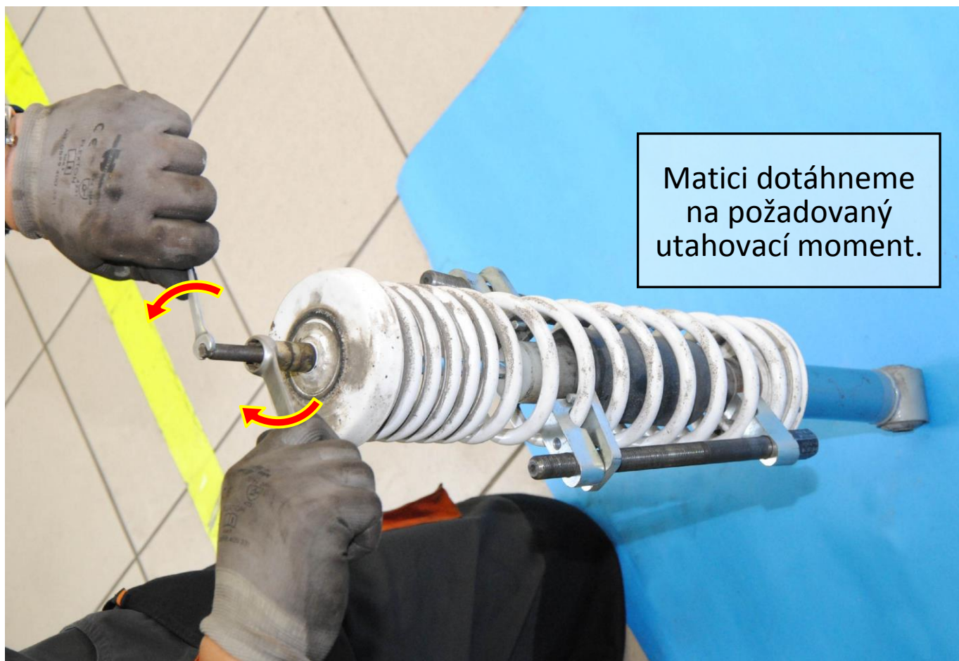
Obr. 18: Montáž tlumiče
