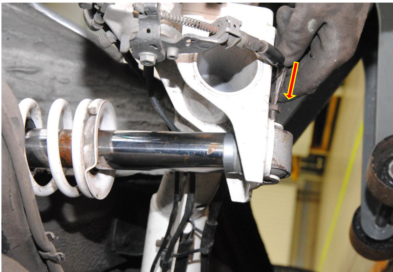
Obr. 23: Zajištění tlumiče
