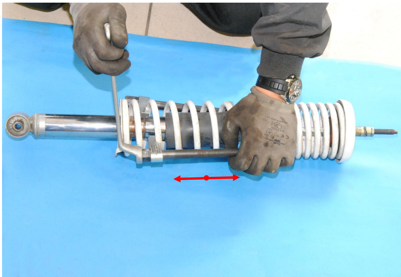
Obr. 19: Demontáž stahováku pružiny
