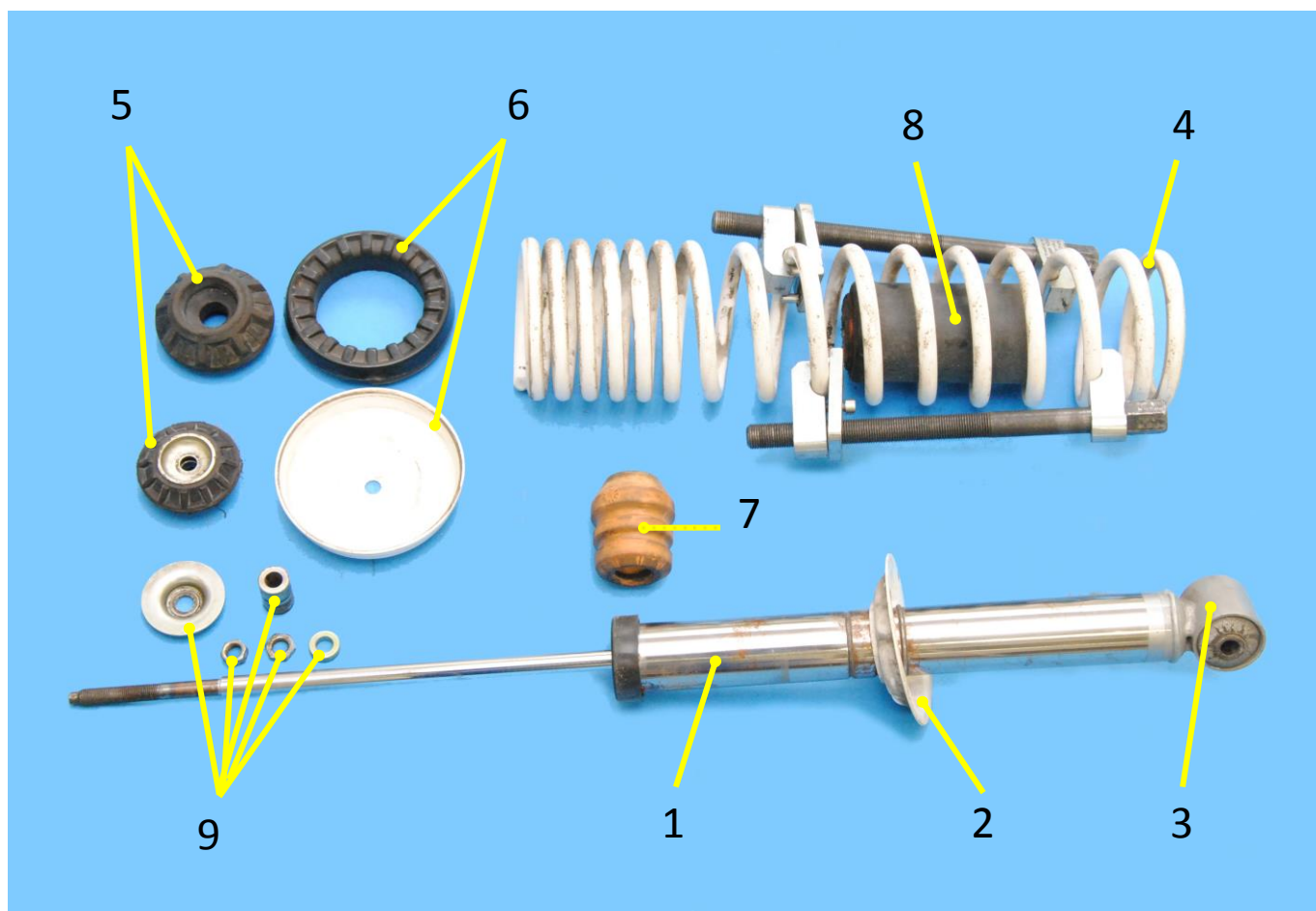
Obr. 15: Hlavní části tlumiče
