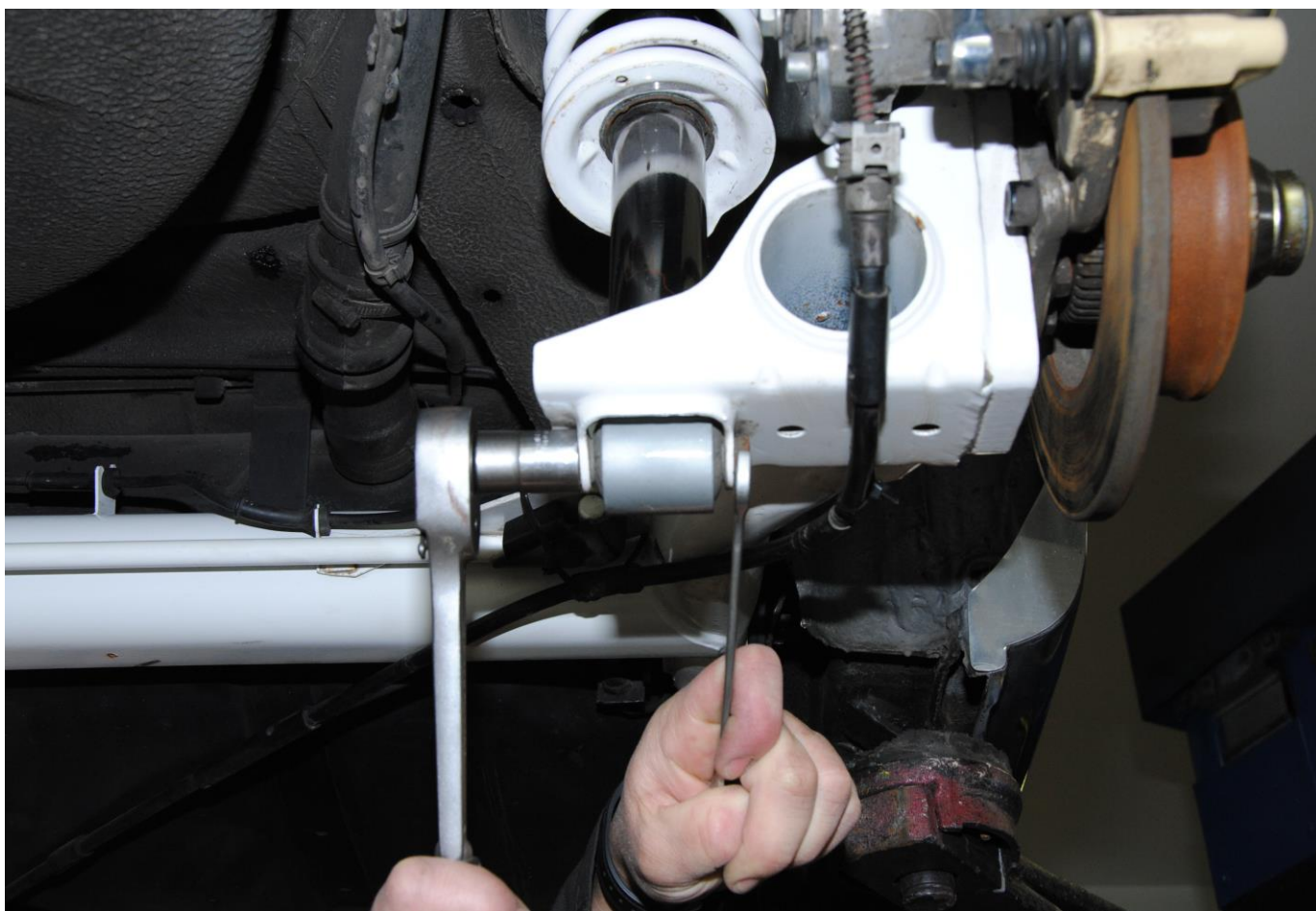
Obr. 7: Povolení zajišťovacího šroubu tlumiče
