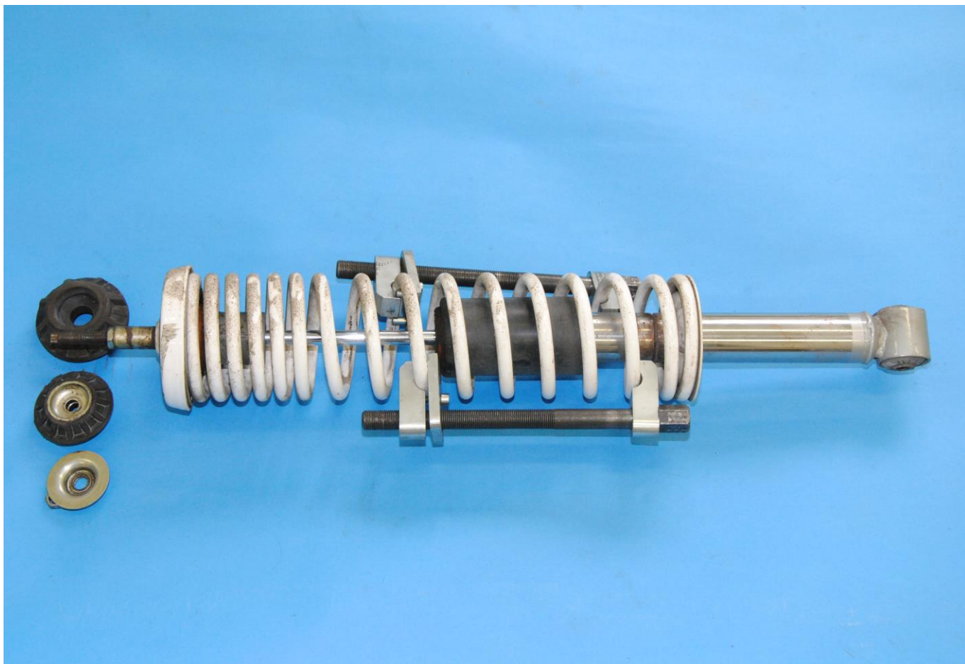
Obr. 12: Stažení pružiny – do uvolnění misek
