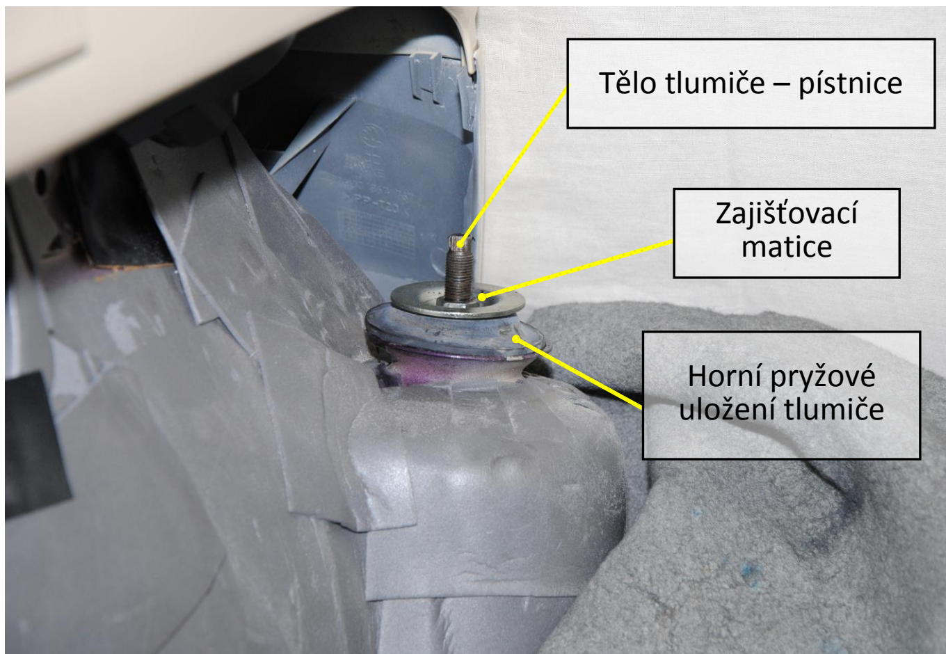
Obr. 3: Horní uložení tlumiče po sejmutí krytu
