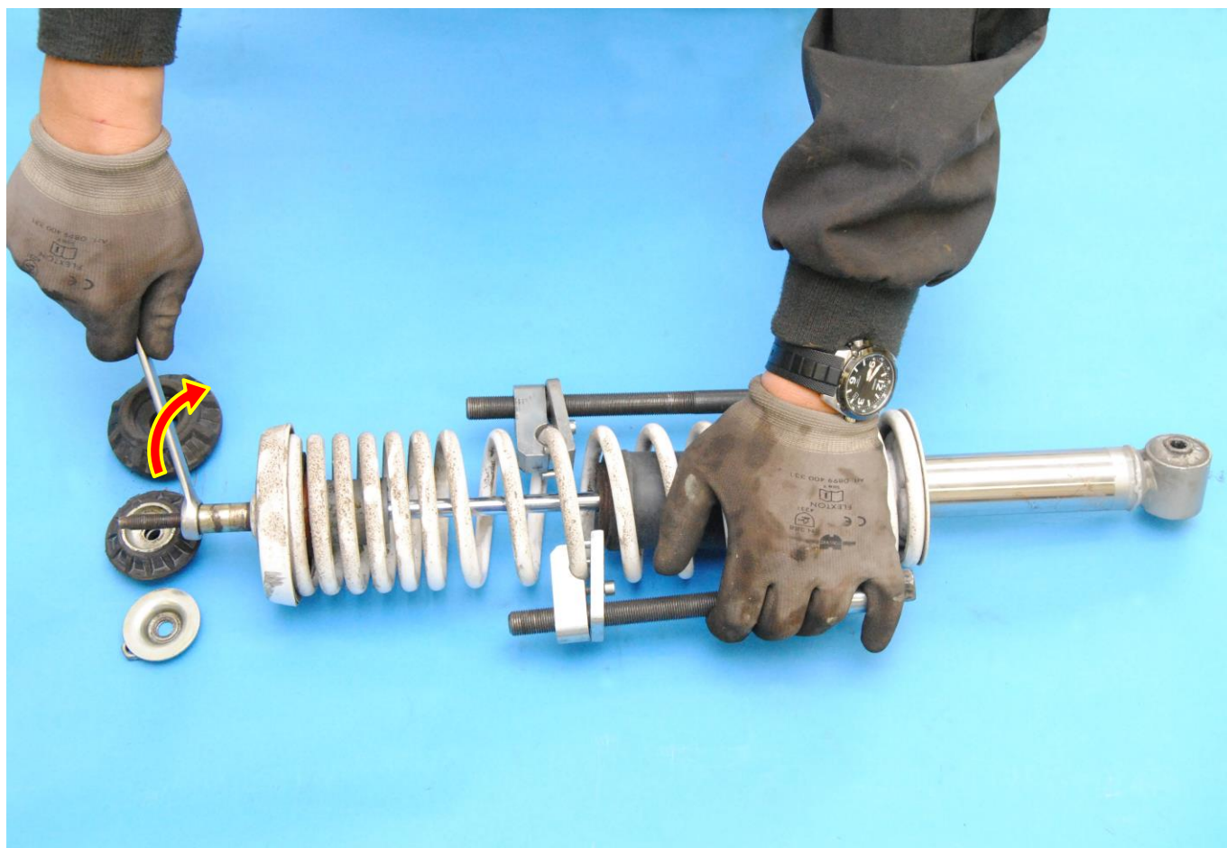
Obr. 13: Demontáž matice zajišťující pístnici
