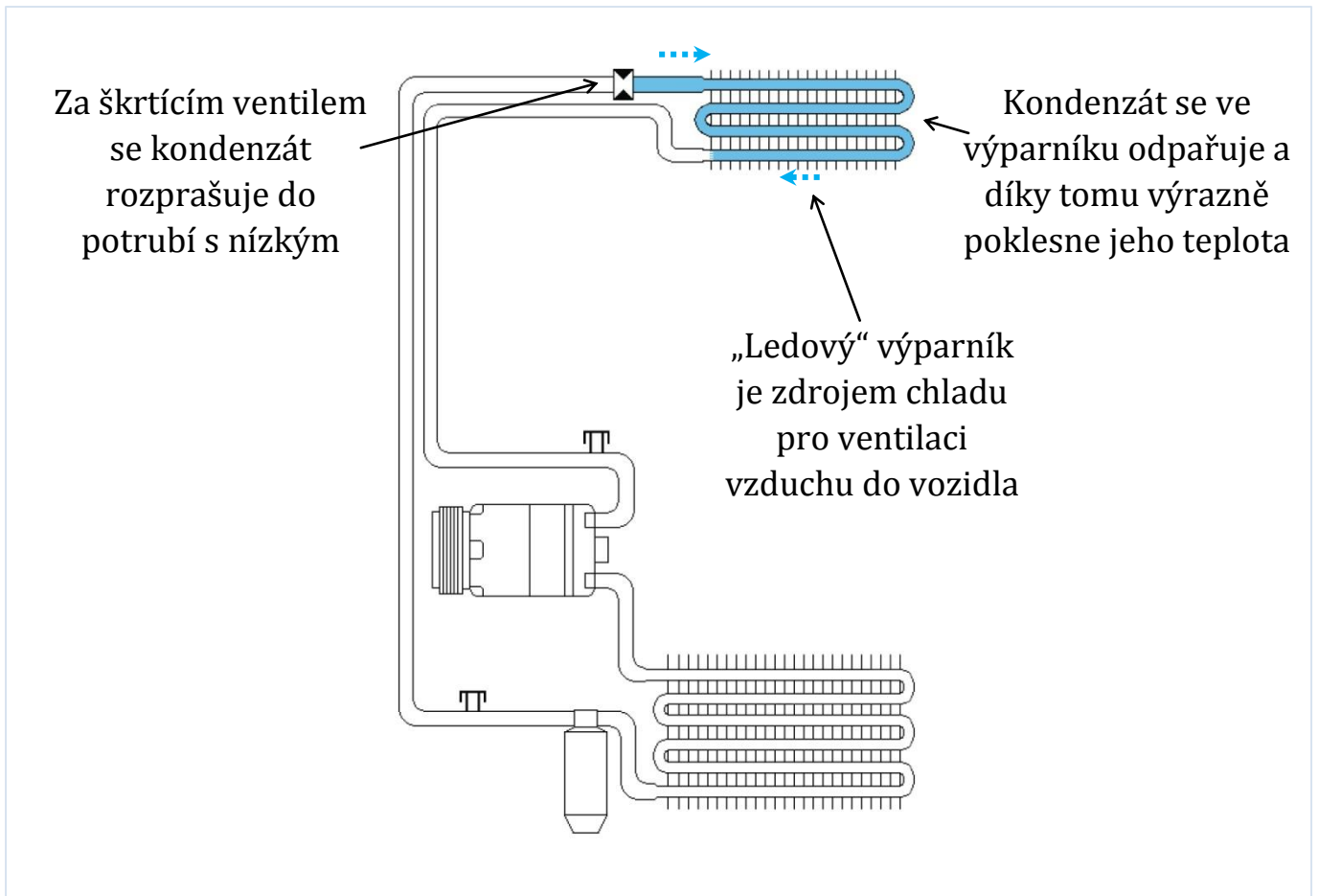
Obr. 7: Odpar kondenzátu ve výparníku
