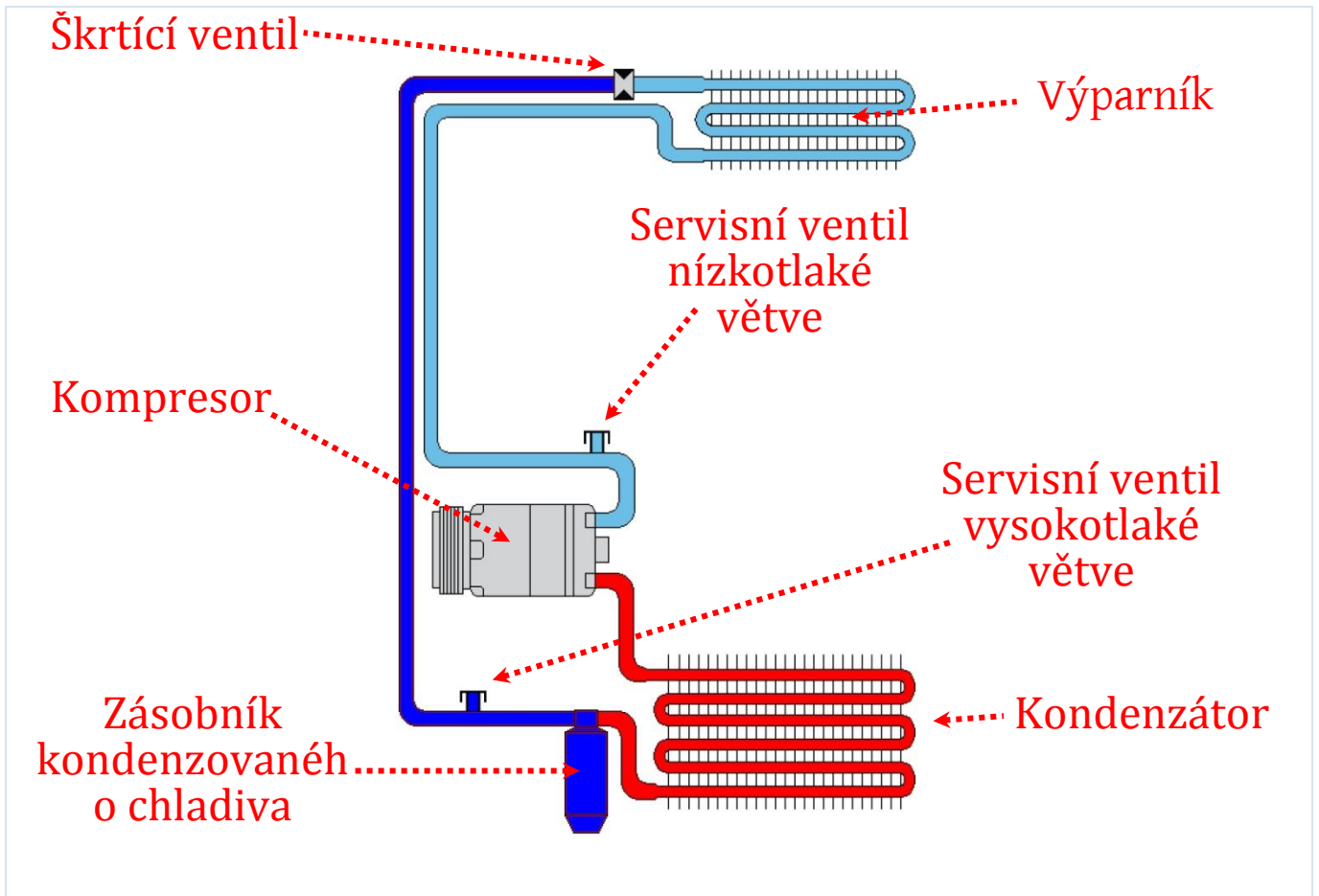
Obr. 2: Schéma klimatizace
