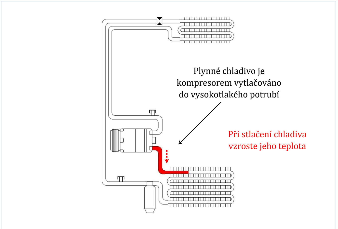
Obr. 4: Komprese chladiva
