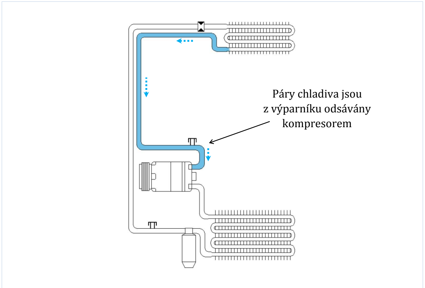
Obr. 8: Doprava par chladiva do kompresoru
