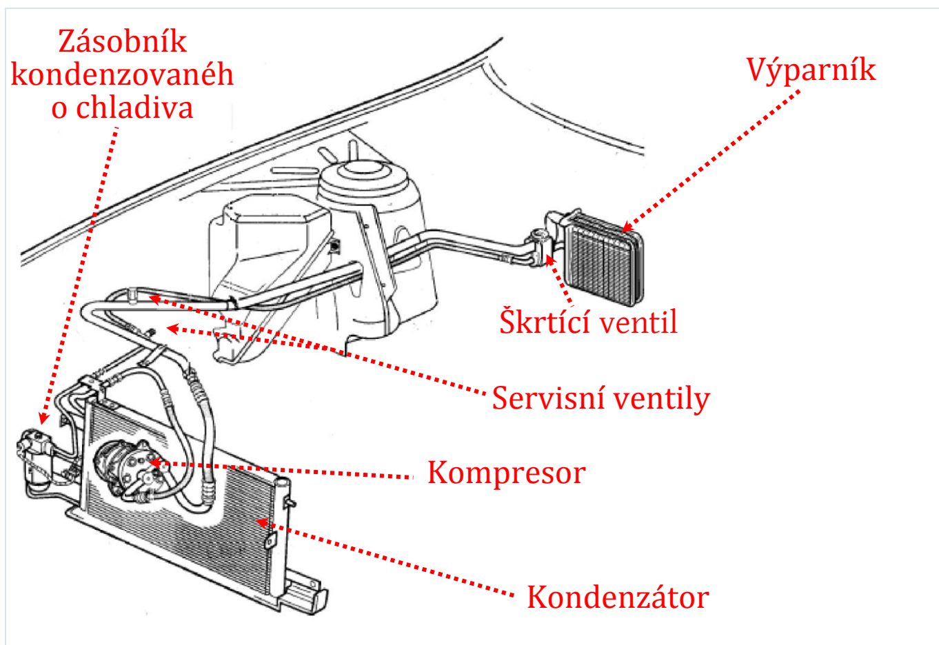
Obr. 1: Rozložení klimatizace pod kapotou vozidla Škoda Felicia
