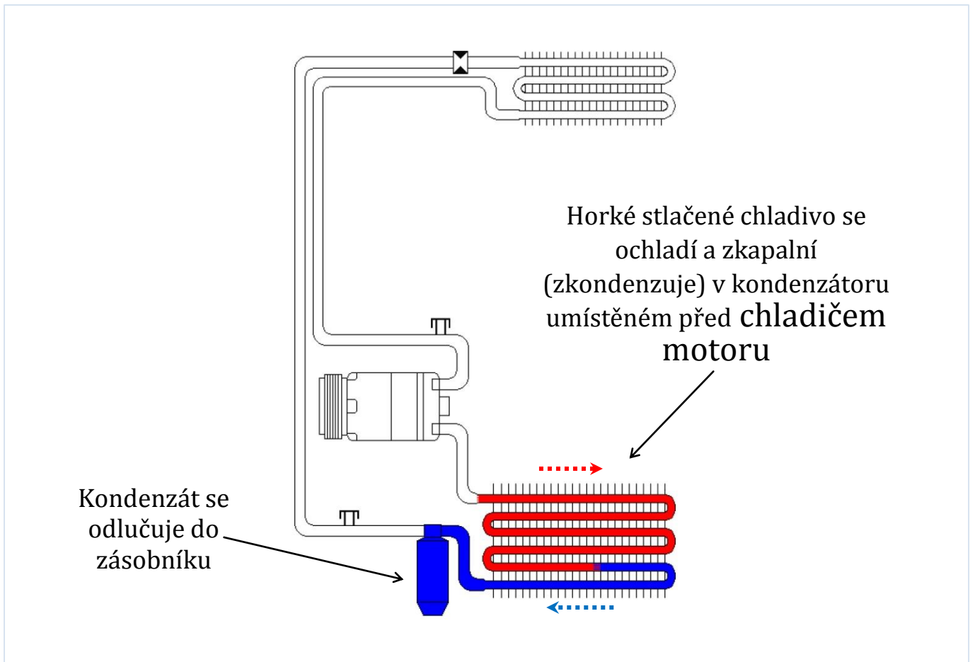
Obr. 5: Chlazení a kondenzace stlačeného chladiva
