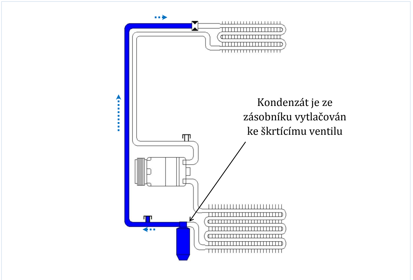
Obr. 6: Doprava kondenzátu ke škrťicímu ventilu
