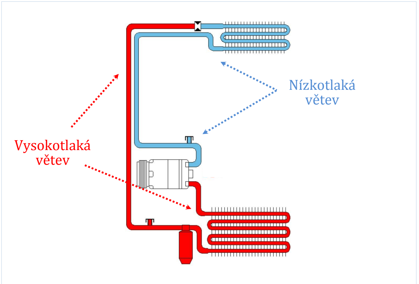
Obr. 3: Větvě klimatizačního okruhu
