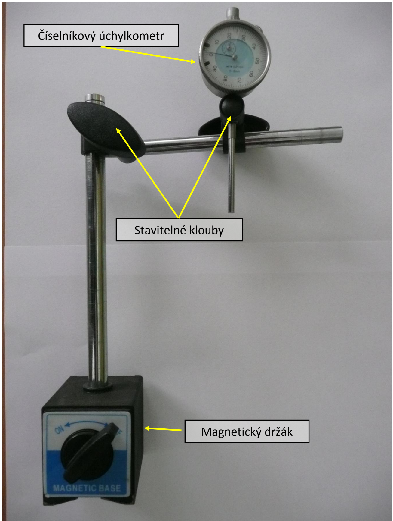
Měřidlo – magnetický stojánek s číselníkovým úchylkoměrem
