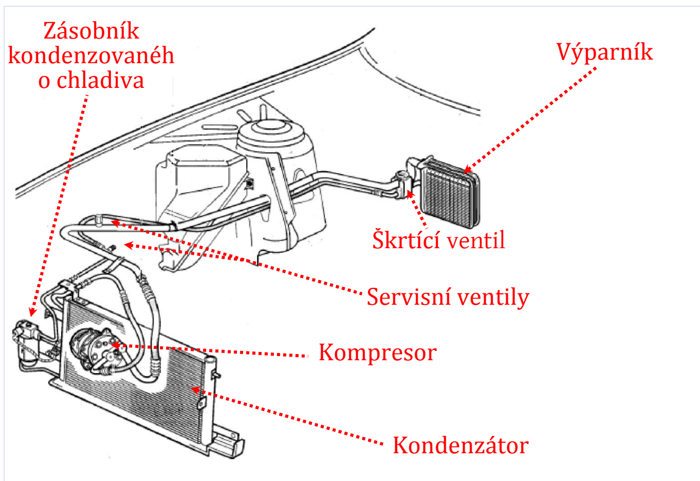
Rozložení klimatizace pod kapotou vozidla Škoda Felicia
