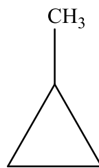
methylcyklopropan
